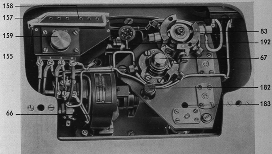
Abb. 7. Kinokammer, Getriebeseite
