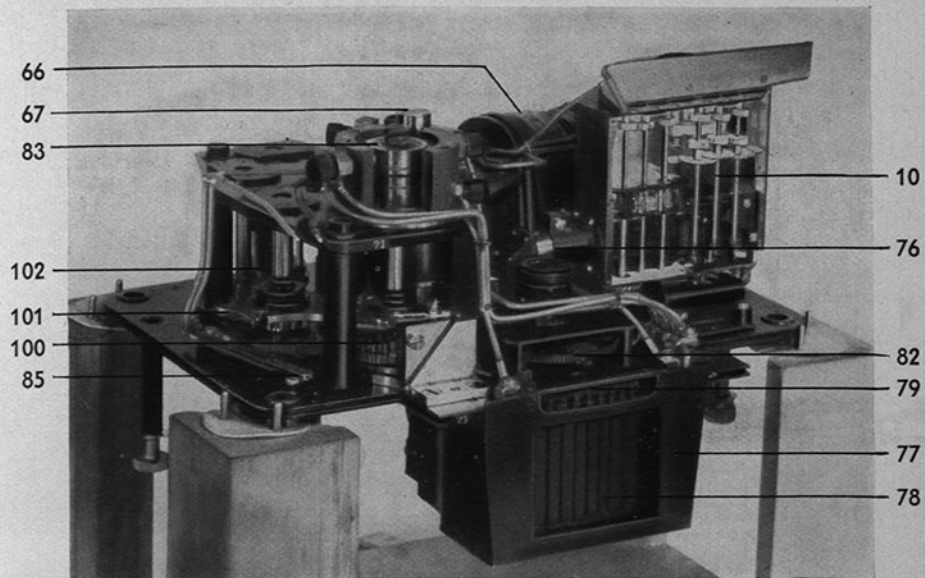
Abb. 6. Kinokammer auf Montagegestell
