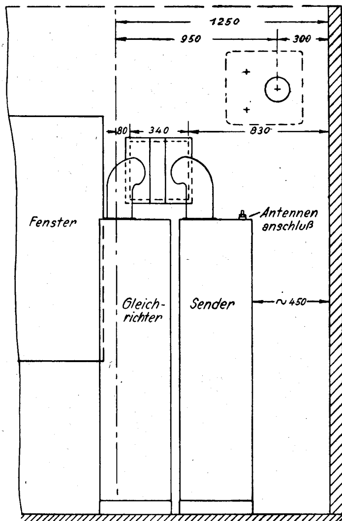
Aufstellung an linker Längswand, Ecke rechts
