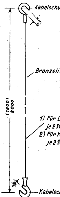
Gegengewichtsanschlußkabel TK 210-1
