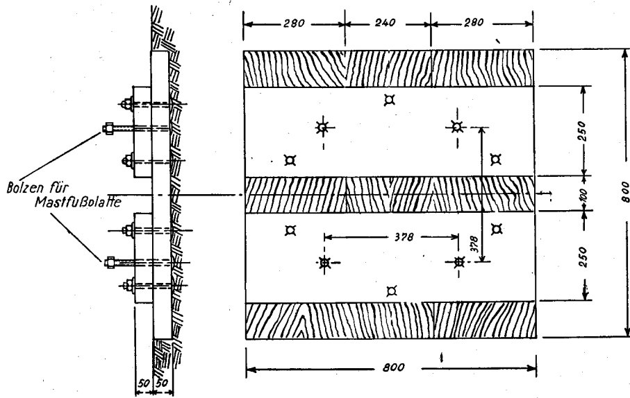
Fundamentplatte aus Holzbohlen
