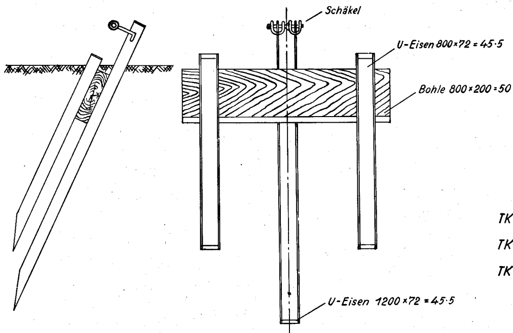
Mastabspannanker
