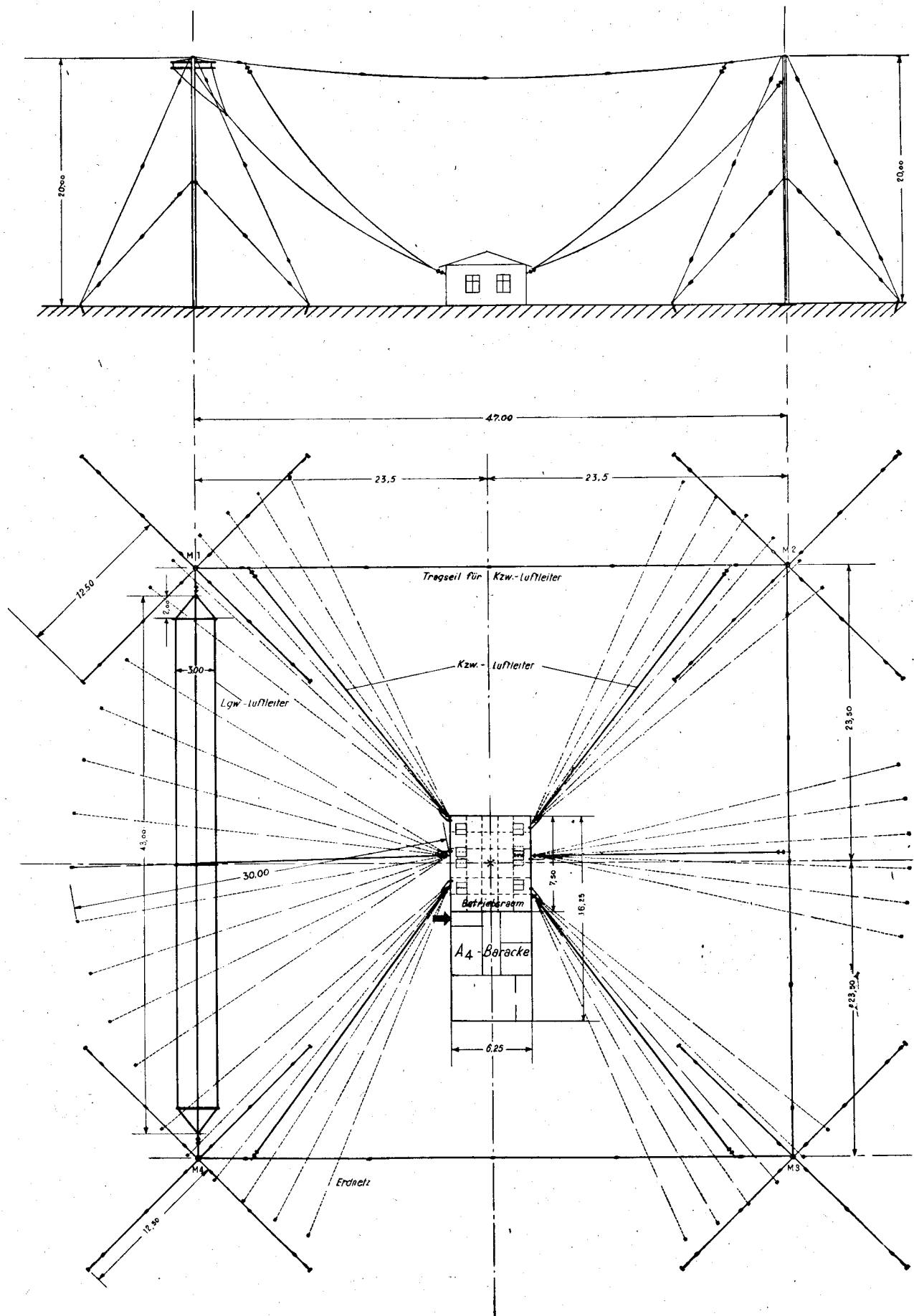
Aufbauplan für FuSZ 3. b. V. (Sonder-Ausführung)
