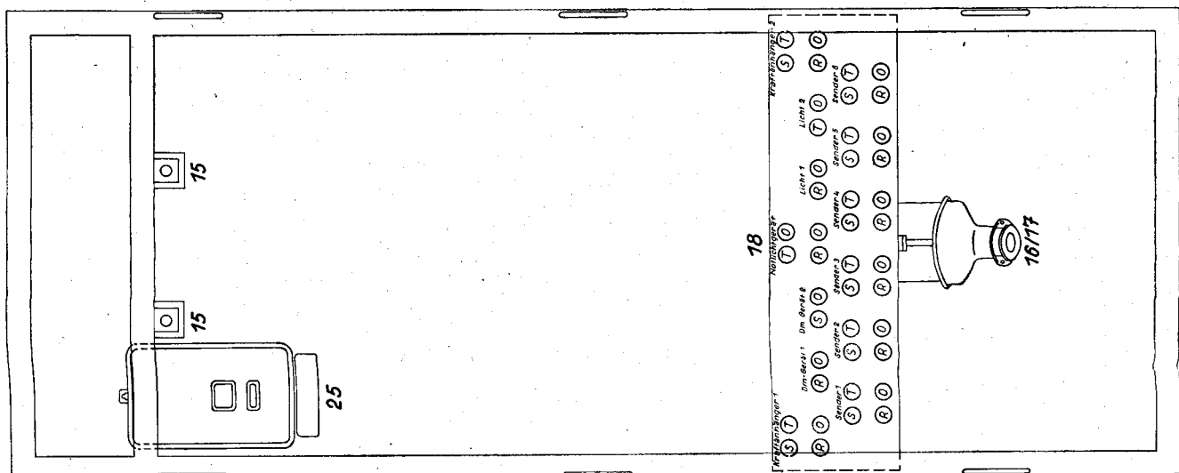
Rückansicht ohne Türen
