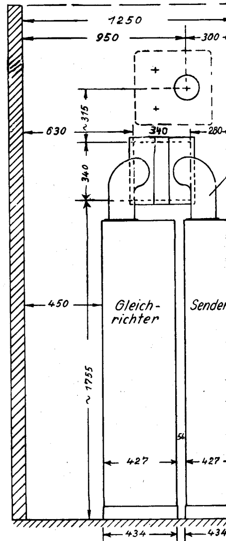
Aufstellung an rechter Längswand
