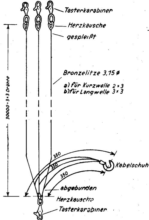
Gegengewichtsdrähte TK 204-1 (Lgw) TK 206-1 206-2 (Kzw)
