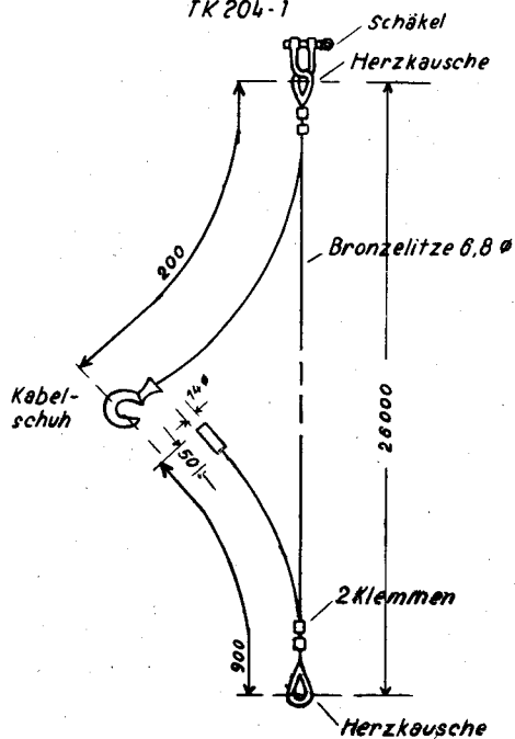
Luftleiterzuleitungsdraht (Lgw) TK 204-1
