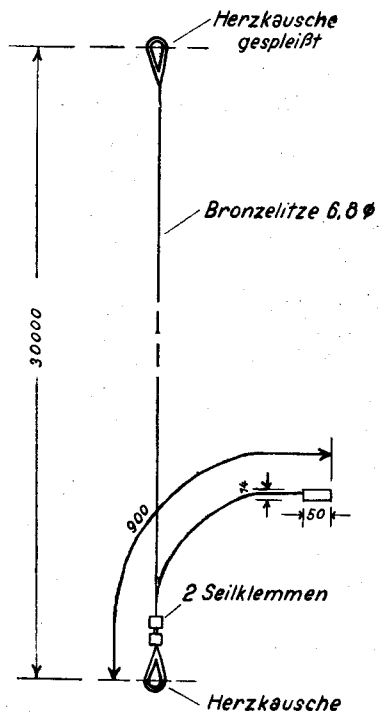
Luftleiterdraht 30m lang TK 206-1 (4) TK 206-2 (2)
