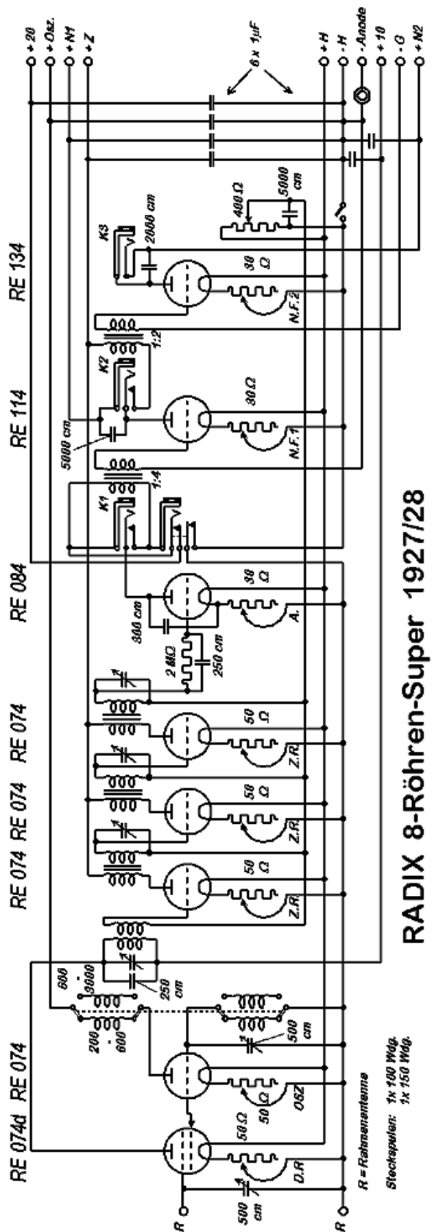
Schaltbild des 8-Röhren-Supers 1927/28 mit unabgeschirmtem ZF-Teil.
