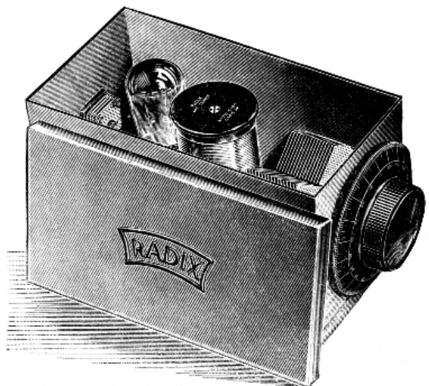
Bild 4: RADIX-HF-Box von 1928 (aus Radio-WEB-Katalog 1927/28).
