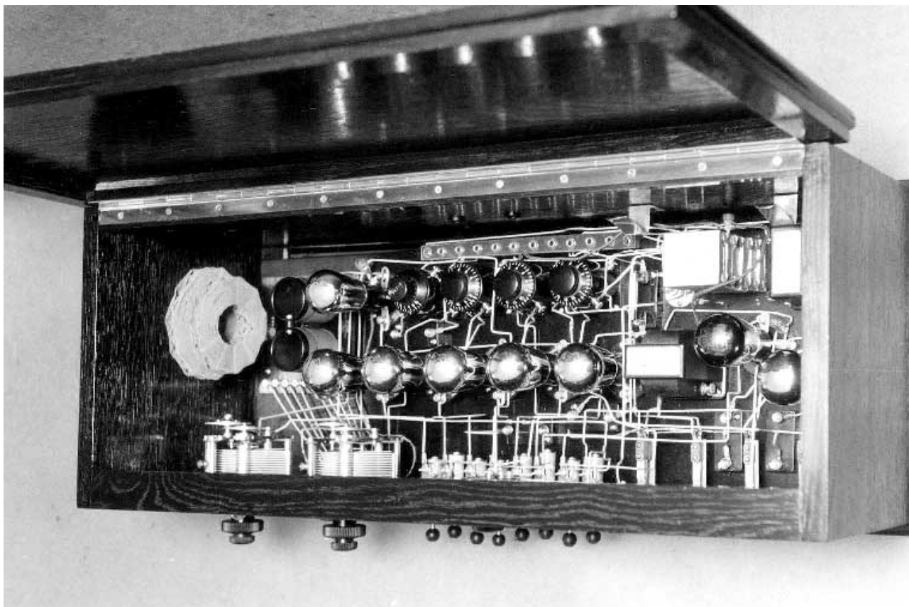
Bild 10: Chassis von oben.
